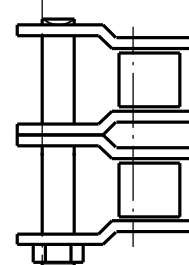
Gekröpftes Glied mit Mutter
